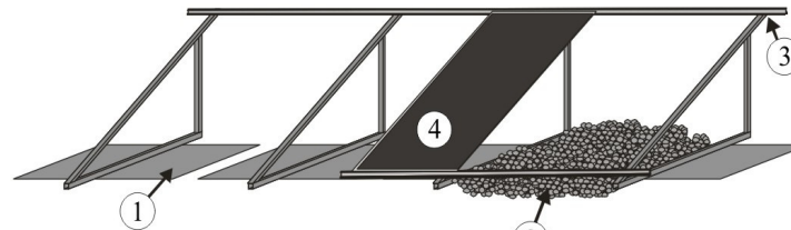
Explosionszeichnung
